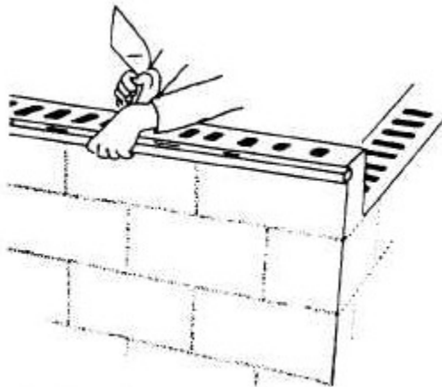
1. Aligning
