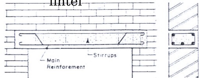
(a) Longitudinal Section
