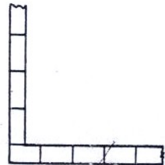
1, 3, 5 --- Courses (d) Plan
