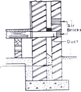
(d) Ventilation Provisions
