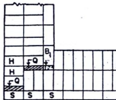
(d) Plan for 2\frac{1}{2} Brick Thick Wall
