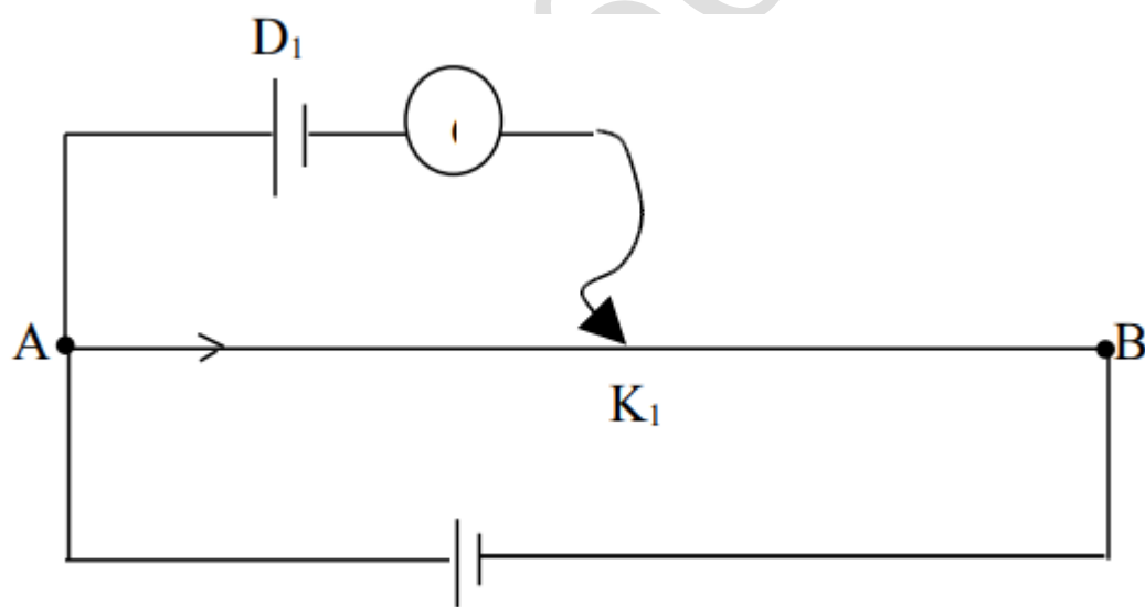
Fig: The Potentiometer
