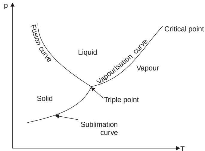
Fig. 7.4. p - T diagram.
