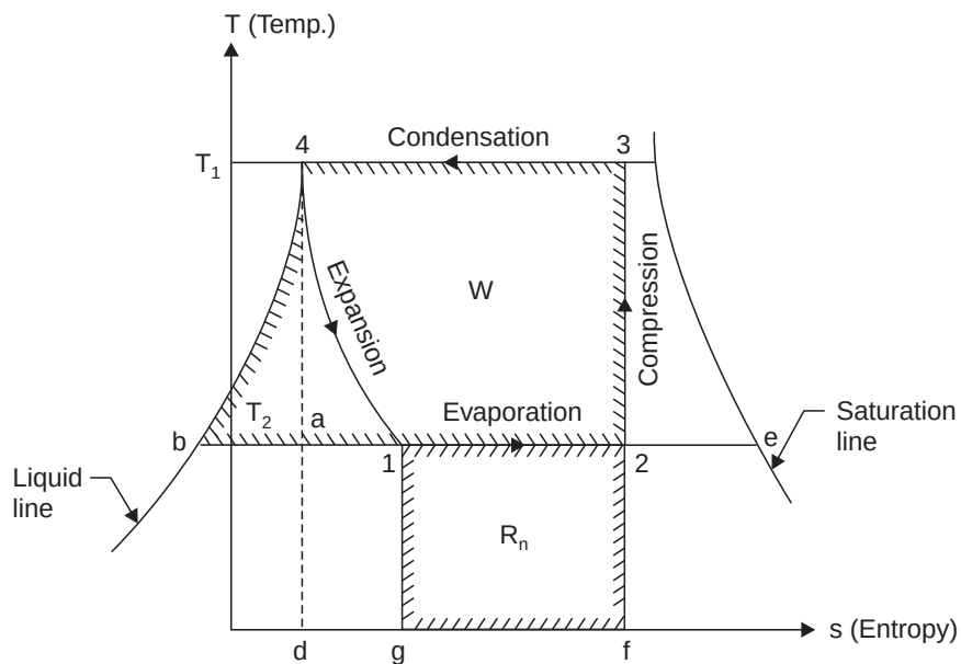
Fig. 14.12. T - s diagram.
