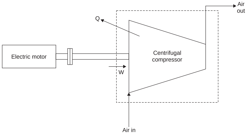
Fig. 4.35. Centrifugal compressor.
