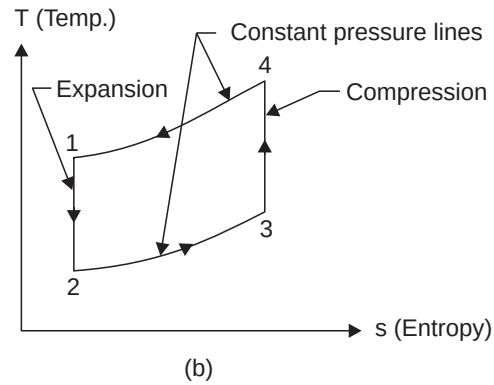
Fig. 14.5. (b) T - s diagram.
