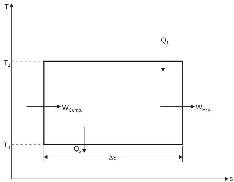
Fig. 6.4. Carnot-cycle.
