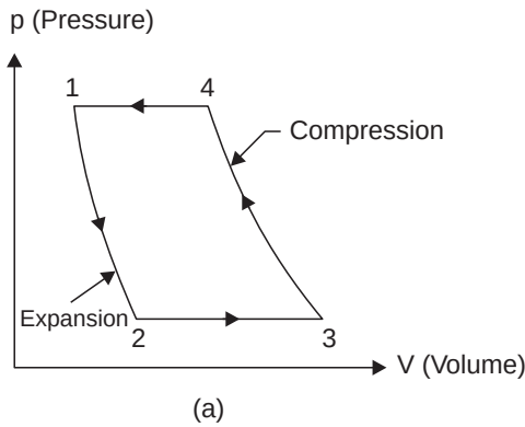
Fig. 14.5. (a) p - V diagram.
