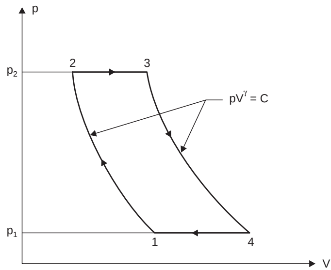
Fig. 13.48. p - V diagram.
