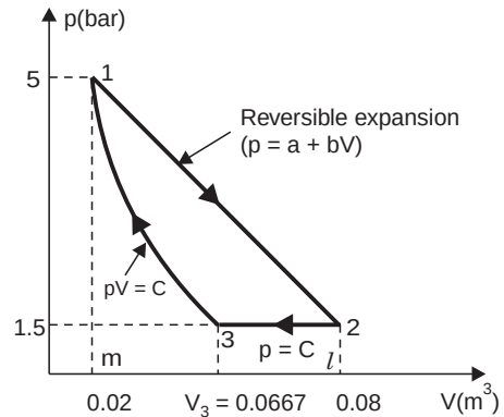
Fig. 4.26. p - V diagram.
