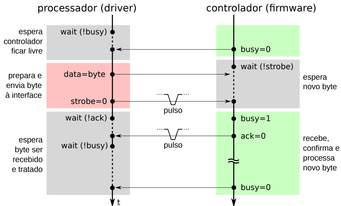
Figura 20.3: Entrada/saída controlada por programa.
