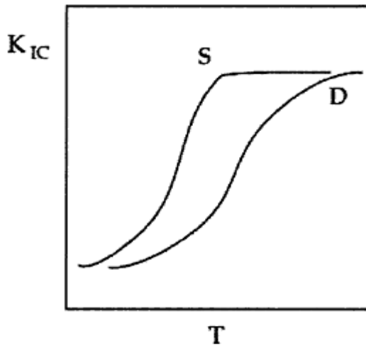
Figure 3-13 Static (S) and Dynamic (D) Fracture Toughness
