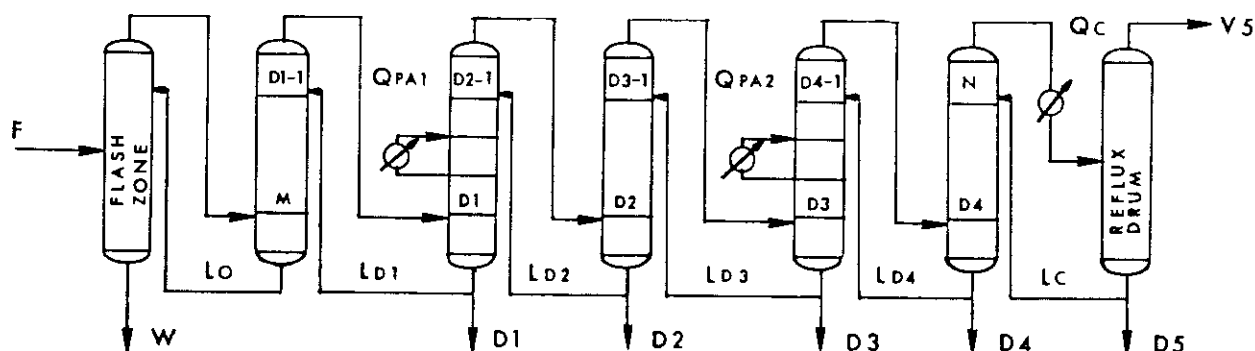
FIG. 2-3c - TYPE A (PUMPAROUND REFLUX)
