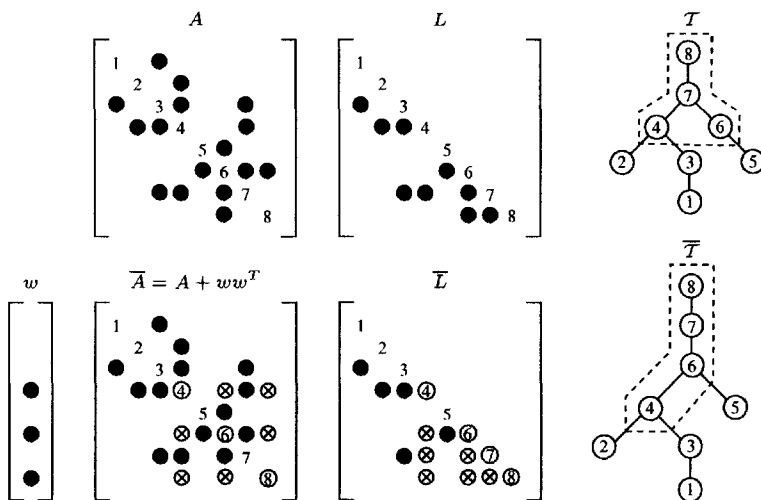
Figure 4.11. Rank-1 update
