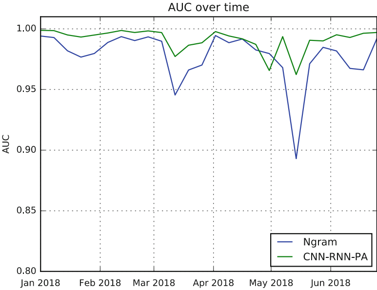
Fig. 5 AUC over time
