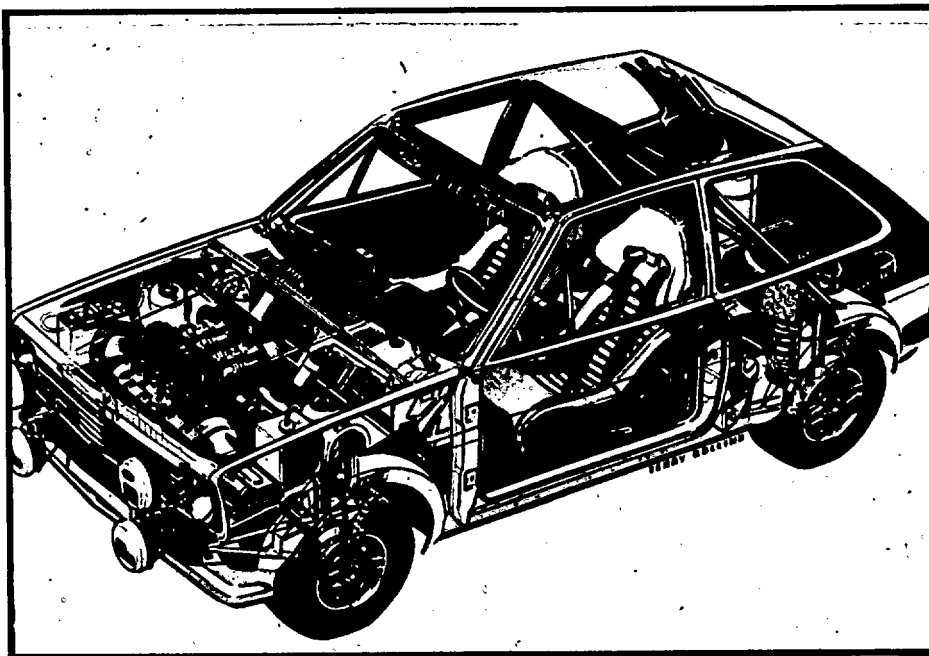
Radiografía del Fiesta 1600, en esta versión de dos carburadores a doble cuerpo, de desarrollo 150 CV aproximadamente.
