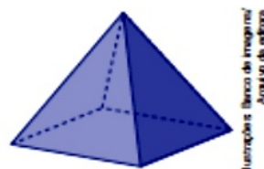
Pirâmide de base quadrada
